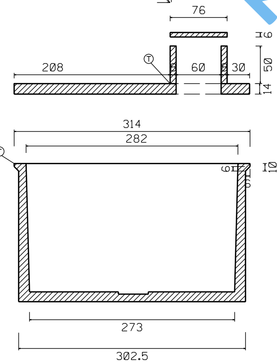
ŘEZ B-B'
