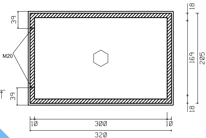
POHLED A-A'
