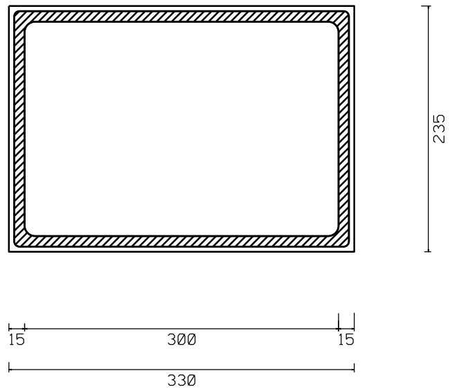
POHLED A-A'
