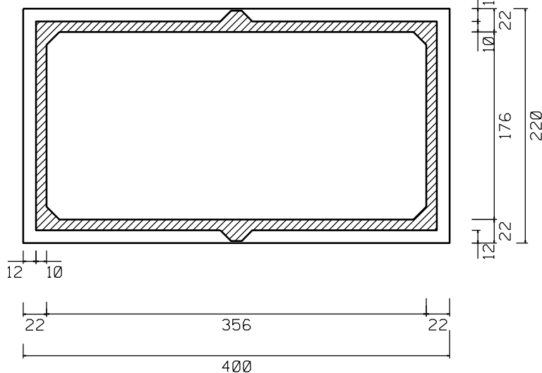
POHLED A-A'
