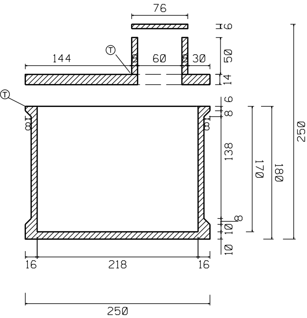
ŘEZ B-B'
