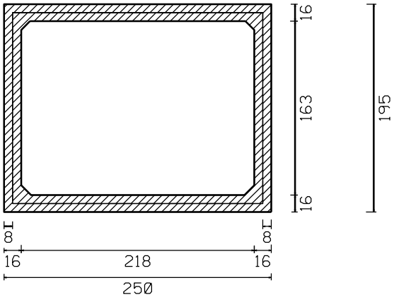
ŘEZ C-C'
