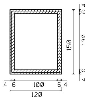
POHLED A-A'
