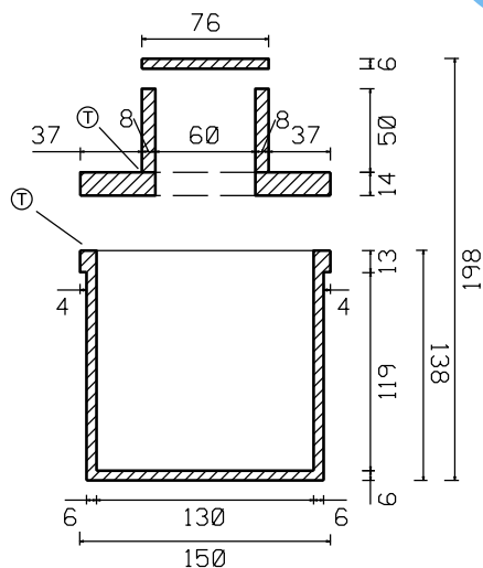
ŘEZ B-B'
